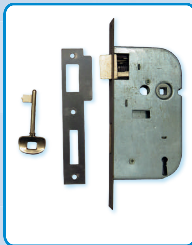
Fechadura "Inferlar"
